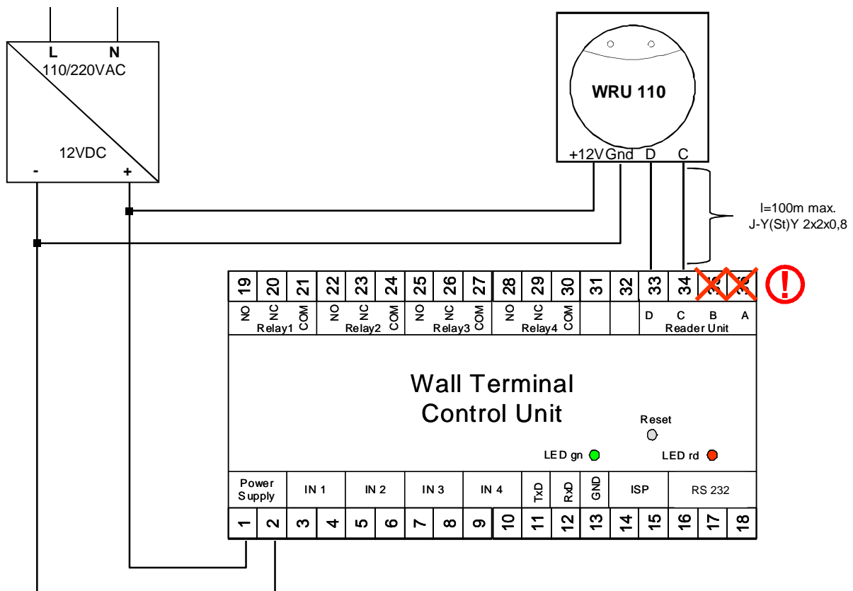
Anschlußschema Wiring Scheme
